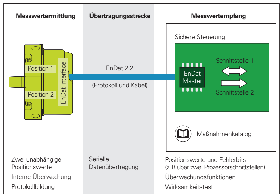
Sicherheitsbezogenes Positionsmesssystem
