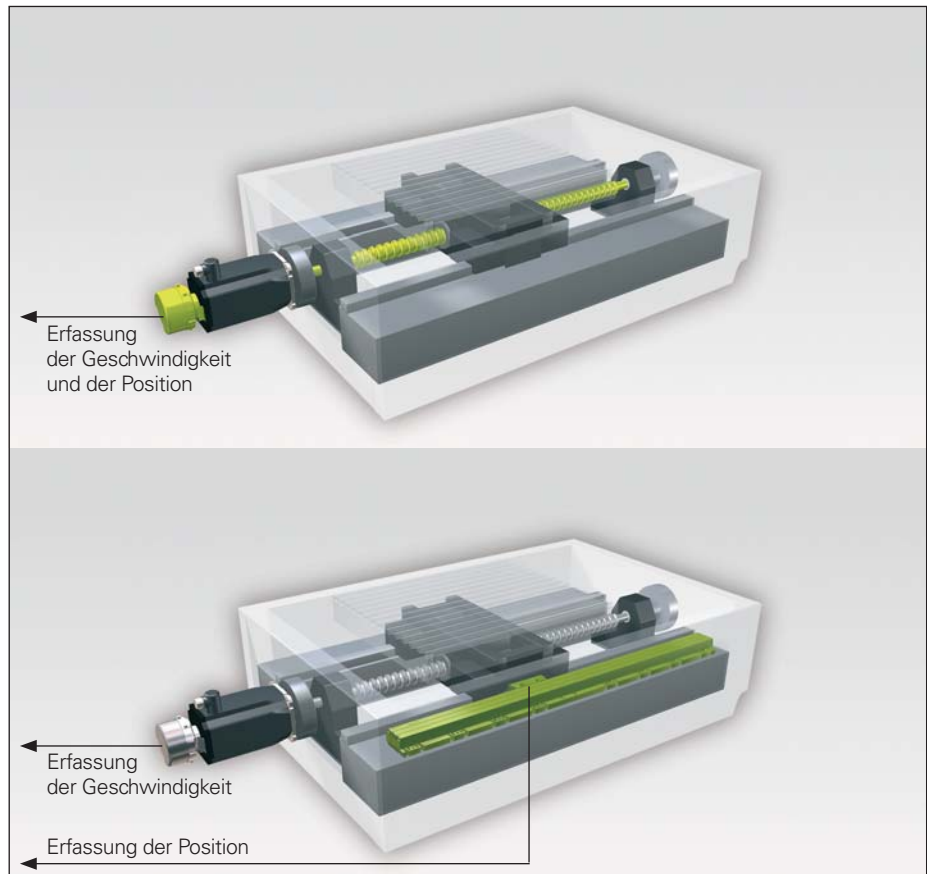
Abbildung 2 Positionsregelung im Semi-Closed Loop (oben) und im Closed Loop (unten)
